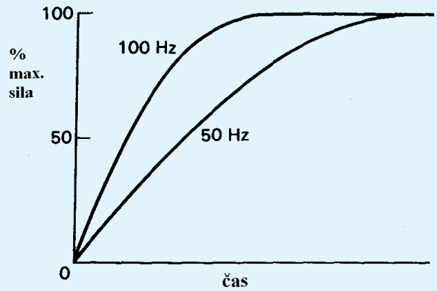
Slika 3: Učinek večje frekvence sproženja akcijskih potencialov na hitrost prirastka sile ob začetku kontrakcije, ki je ob večji frekvenci (100 Hz) večja kot pri nižji (50 Hz) (Komi, 1992).
