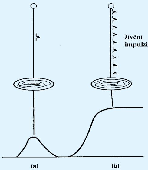
Slika 2: Učinek frekvence sproženja akcijskih potencialov na mišično silo: (a) pri enem akcijskem potencialu je odziv kratek, sila pa je majhna in (b) pri več zaporednih akcijskih potencialih je sila večja in traja dlje (Komi, 1992).
