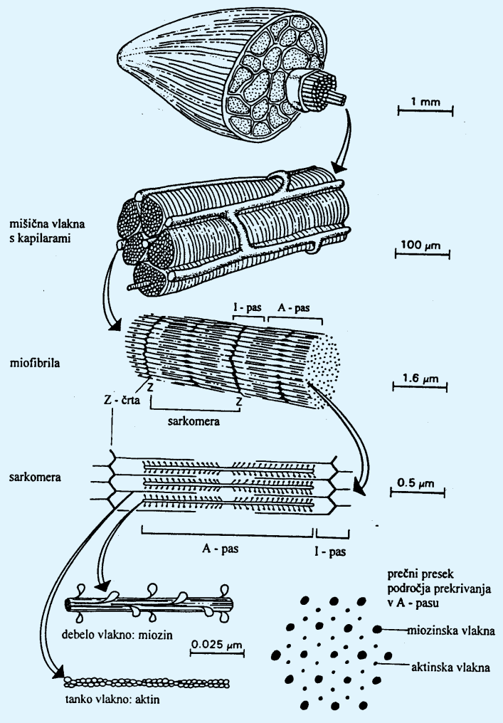
Slika 1: Prikaz strukture skeletne mišice od mišičnega vlakna do sarkomere (Di Prampero, 1985).
